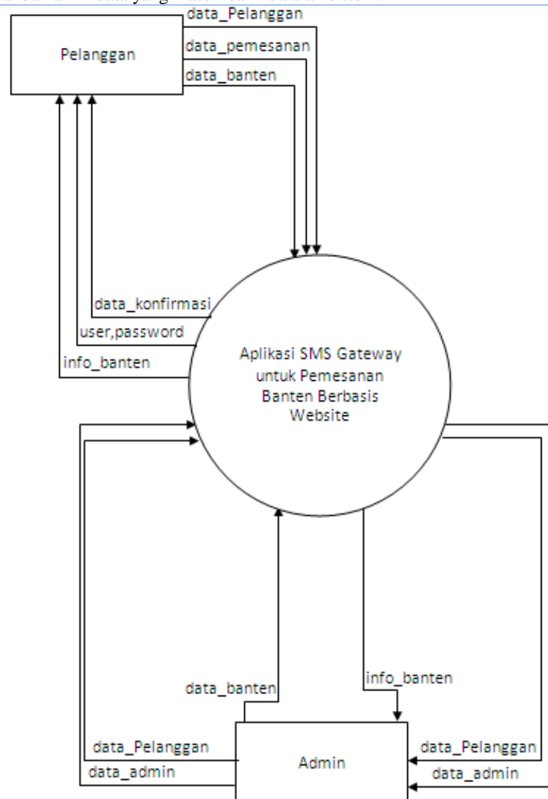
Gambar 3 Diagram Konteks
