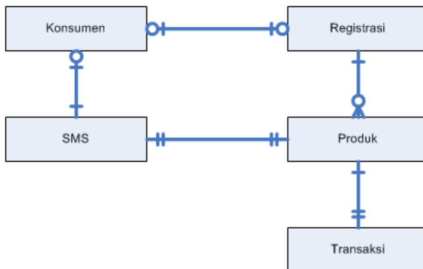
Gambar 7 ERD
