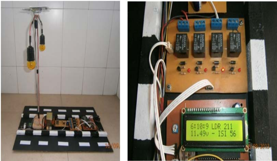
Gambar 7. Keseluruhan dari Hardware
